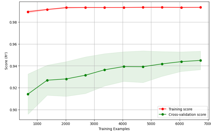
Gambar 7. Grafik Learning Curve( R^2 Score) sebelum Augmentasi Data.
