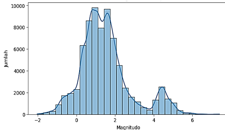
Gambar 3. Distribusi Magnitudo Gempa
