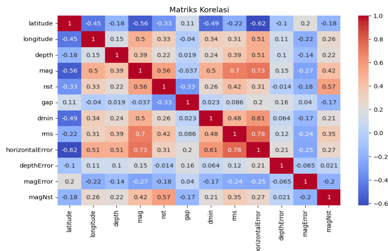
Gambar 5. Hasil Analisis Korelasi antar Atribut
